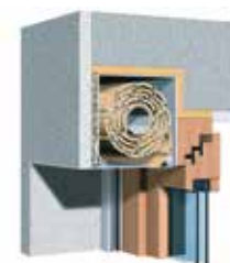
Putzträger-Variante Hinter dem Putz – nahezu unsichtbar.
