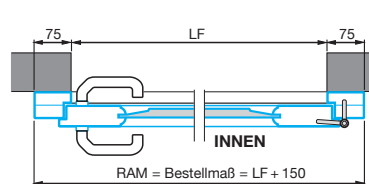
Holz-Nebentür Einbau hinter der Öffnung
