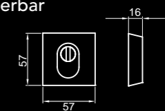
Schutzrosette – ESR 550 Q KS ES1 nach DIN 18257
