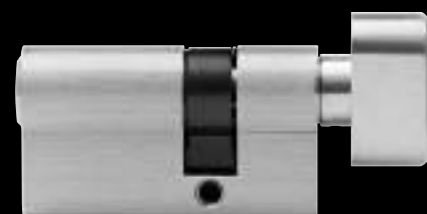
Knaufzylinder für Glastürschloss ZEGS KZA 35/20 (Knebelseite 20 mm) ZEGS KZB 20/35 (Knebelseite 35 mm) Farbe: Nickelmatt
