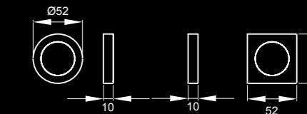
Blindrosette Rund : EZ 1332 BL Quadratisch : EZ1340 BL Farbe: Edelstahl matt
