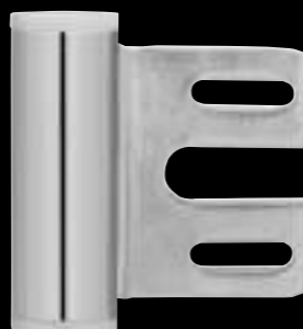
Rahmenteile – EGB 3 V 8000 WF für Metall- bzw. Objektzargen, Höhe: 48,5 mm Farbe: Stahl verzinkt
