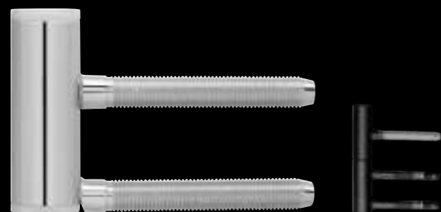
Rahmenteile – EGB 3 V 4400 WF für Holzzargen, Höhe: 48,5 mm Farbe: Stahl verzinkt, Antik Bonze Optik/Kosmos Schwarz*
