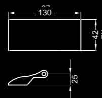
Glasstürband 2-teilig – EGB 102 Farbe: Edelstahl matt
