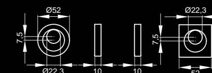
Blindrosette Rund : EZ 1332 BL Quadratisch : EZ1340 BL Farbe: Edelstahl matt
